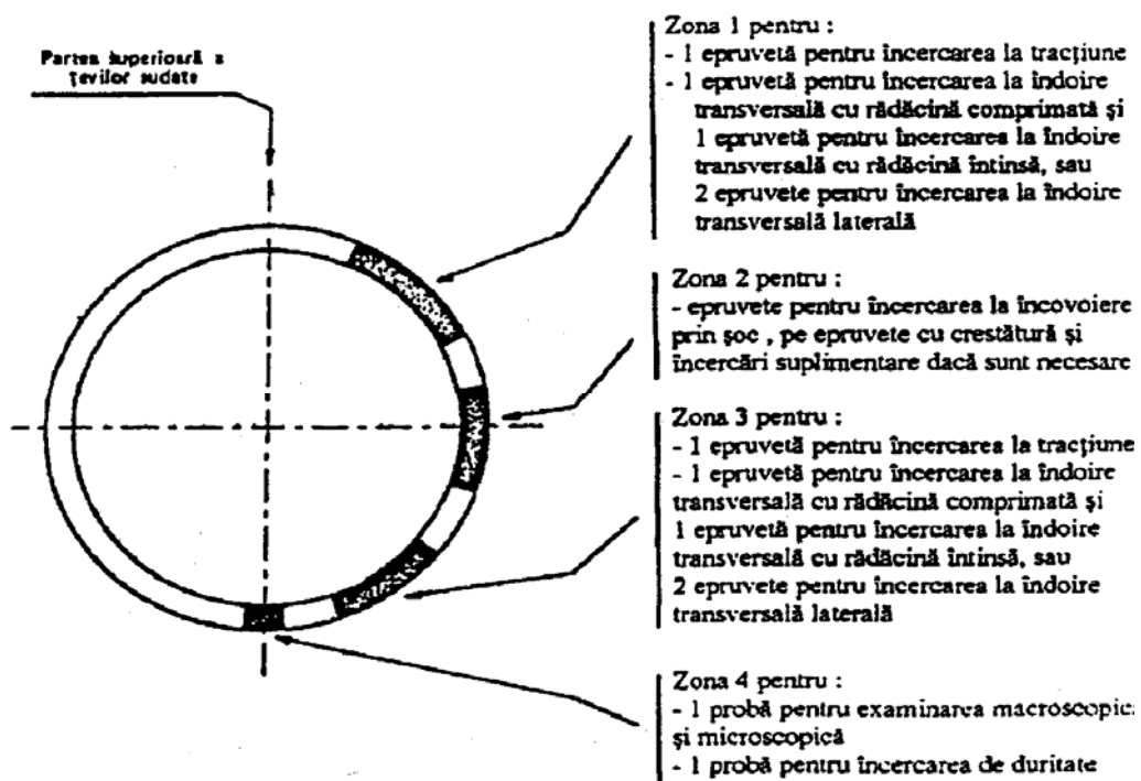
Figura 7 - Localizarea epruvetelor pentru o sudură cap la cap la țevi
